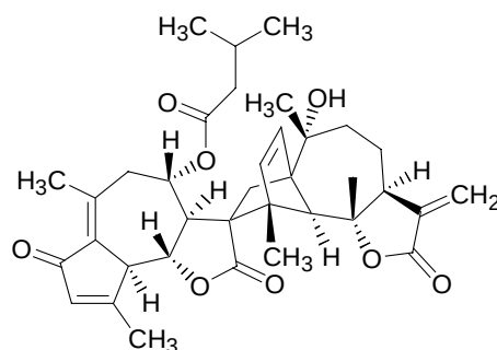
Schéma 4 : Structure de l'artémínolide
