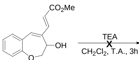
Schéma 163 : Essai d'isomérisation en conditions basiques
