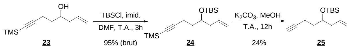
Schéma 111 : Préparation de l'ényne 25
