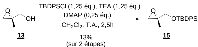
Schéma 35 : Silylation de l'époxyalcool 13
