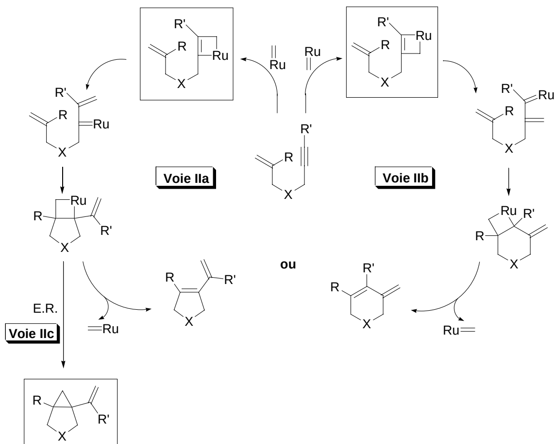
Schéma 79 : Régiochimie de la fixation du ruthénium sur l'alcyne
