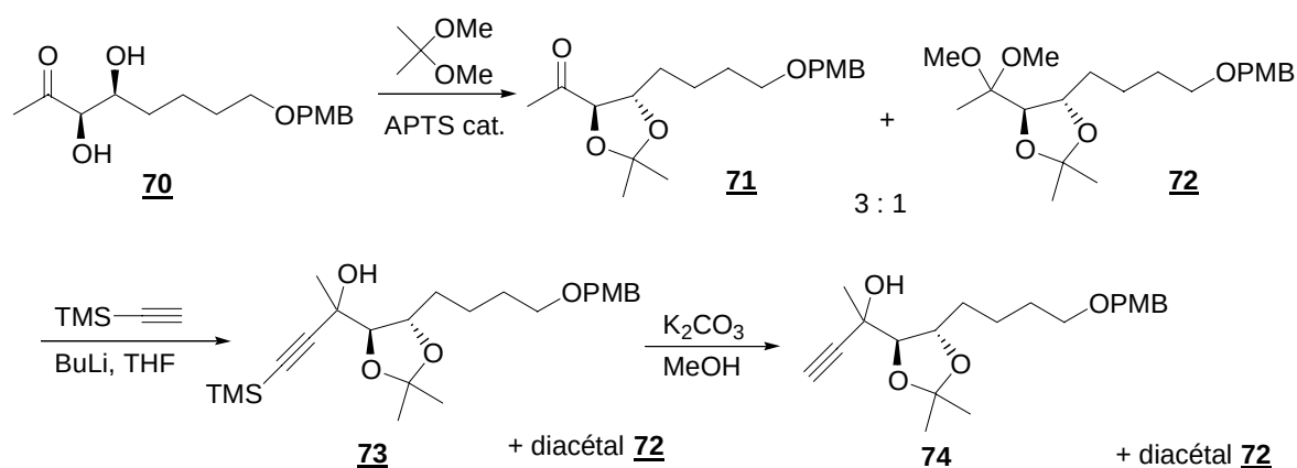
Schéma 169 : Acétalisation du diol 70
