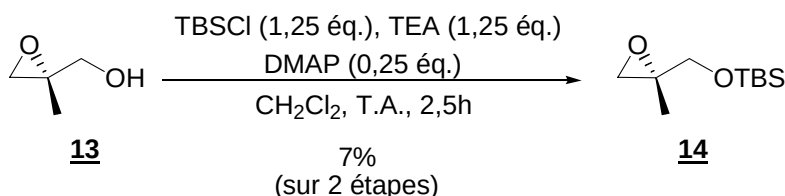
Schéma 34 : Silylation de l'époxyalcool 13
