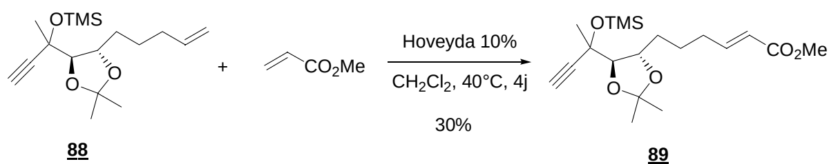
Schéma 184 : Réaction de métathèse de l'ényne 88
