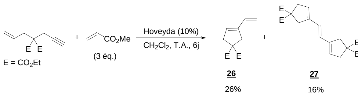
Schéma 113 : Métathèse d'un ényne gem -disubstitué par des groupements esters
