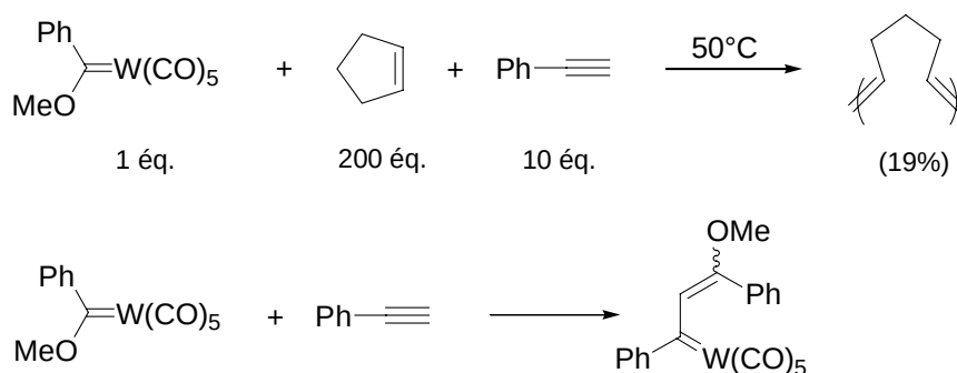
Schéma 59 : Travaux de Katz sur la ROMP
