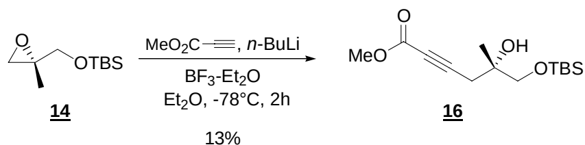
Schéma 36 : Ouverture de l'époxyde 14 par le propiolate de méthyle
