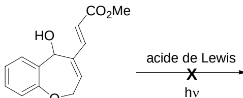
Schéma 164 : Isomérisation sous irradiation photochimique
