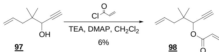
Schéma 196 : Préparation du diényne 98
