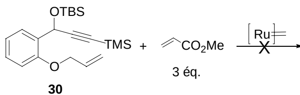
Schéma 124 : Essai de métathèse de l'ényne silylé 30
