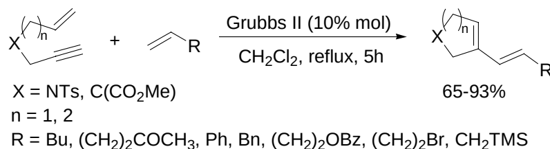
Schéma 148 : Travaux de Lee
