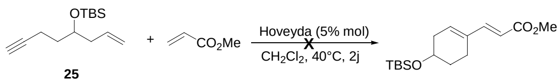
Schéma 112 : Essai de métathèse tandem
