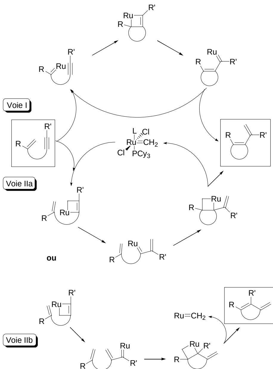
Schéma 73 : Différents mécanismes envisageables pour la métathèse ényne
