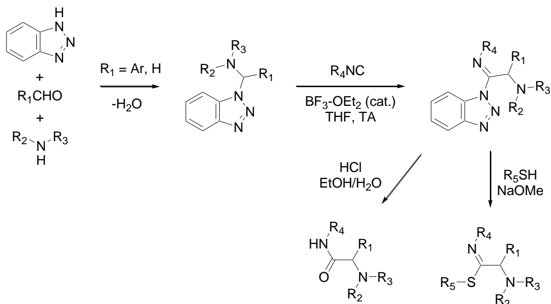
Schéma III.18 : Synthèse de \alpha -aminothioacetimidates et de \alpha -aminoamides par action d'un isonitrile sur un 1-imidoylebenzotriazole.
