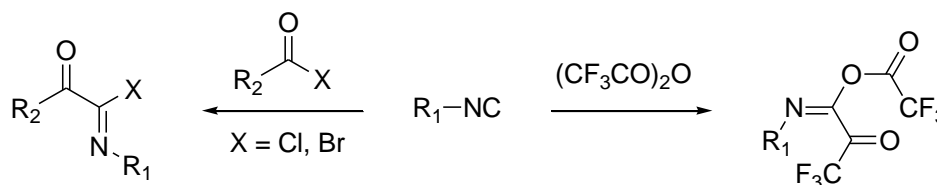
Schéma III.7 : Différents partenaires possibles pour la réaction de Nef.
