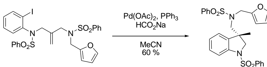
Schéma V.27 : L'emploi de formate de sodium conduit un produit de monocyclisation.
