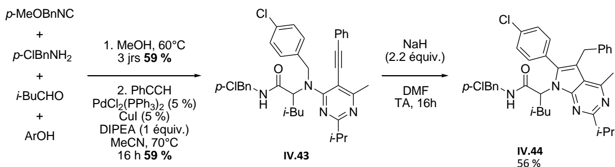
Sch\u00e9ma IV.32 : Nouveau d\u00e9riv\u00e9 de pyrrolo[2,3-d]pyrimidine obtenu dans le cas des ald\u00e9hyles aliphatiques.
