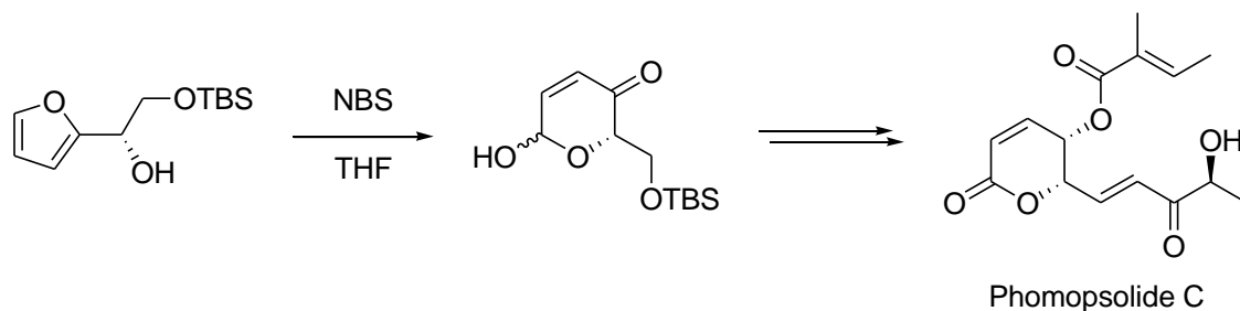
Schéma V.7 : Synthèse énantiosélective d'une lactone \alpha,\beta -insaturée par la réaction de Achmatowicz.
