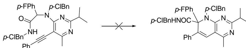
Schéma IV.21 : Produit de cyclisation 6-endo.
