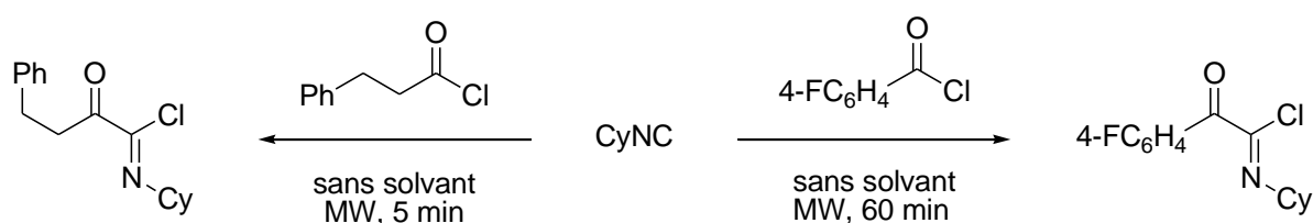
Schéma III.24 : Deuxième stratégie pour le couplage 3-composants.
