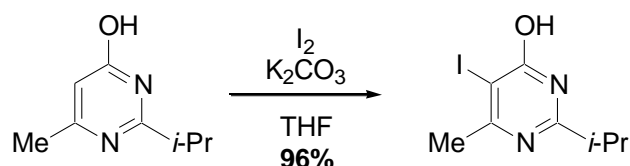
Schéma IV.13: Synthèse d'iodyrimidin-4-ol.
