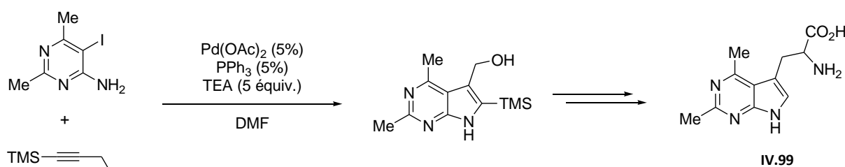
Schéma IV.53 : Synthèse d'analogues de tryptophane.
