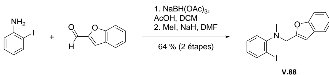
Schéma V.54 : Préparation de la N -méthyl- N -benzofurfurylaniline.
